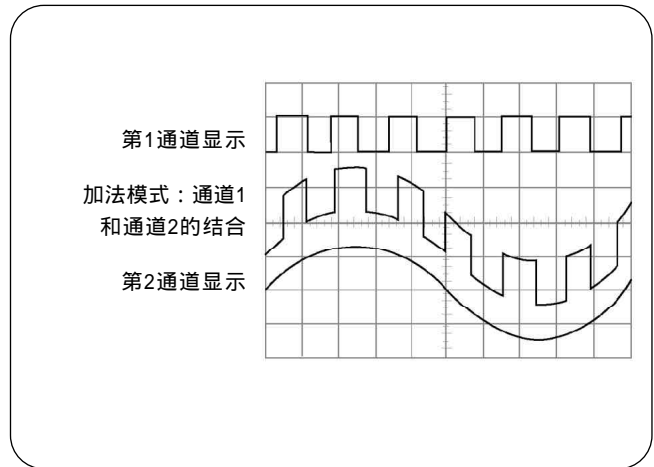
► 图 39. 通道相加
