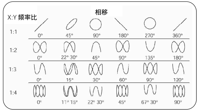
图 70. 李萨如模式
