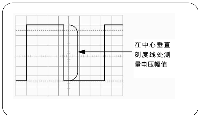
► 图 67. 在中心垂直刻度线处测量电压
