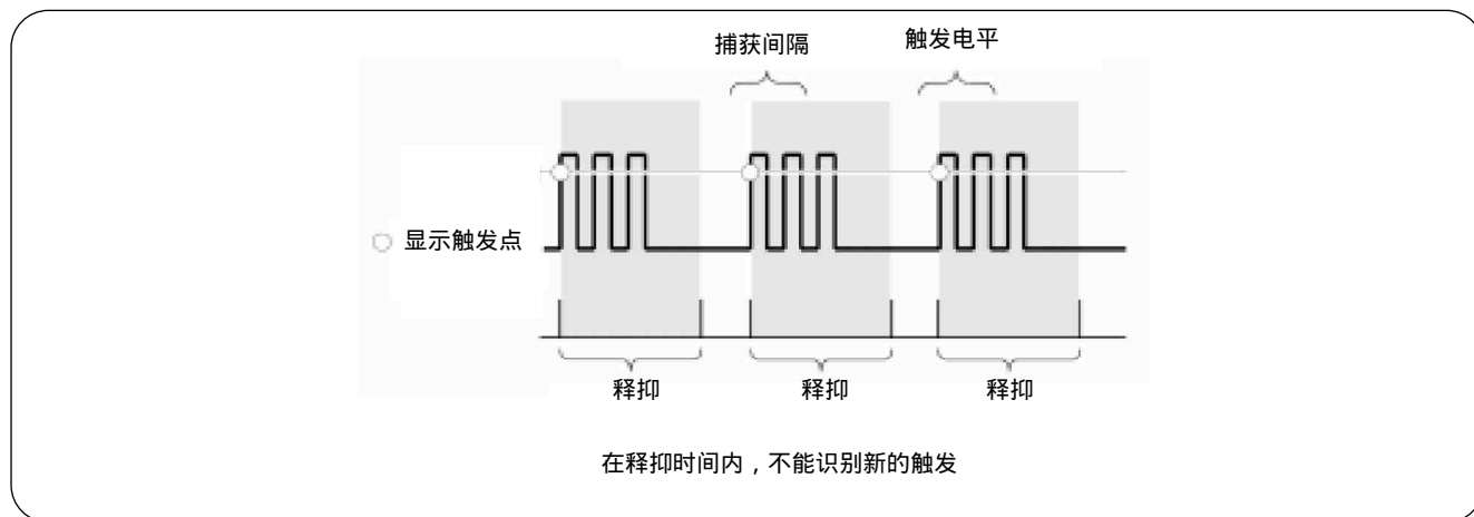
► 图37. 触发释抑
