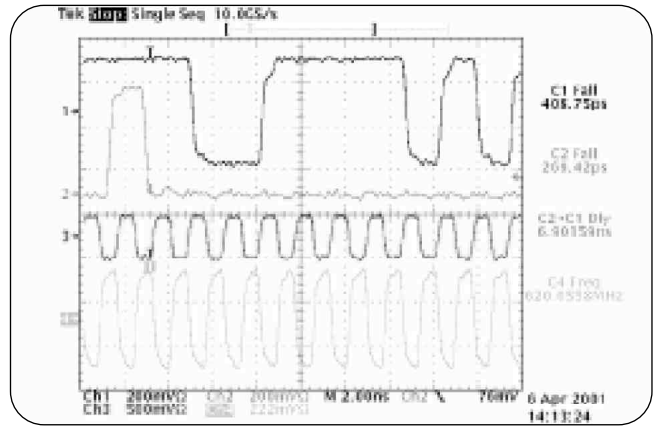
► 图 17. TDS694C 提供多通道同时的高速单次脉冲捕获，增加了对偶发毛刺和瞬态现象的捕获
