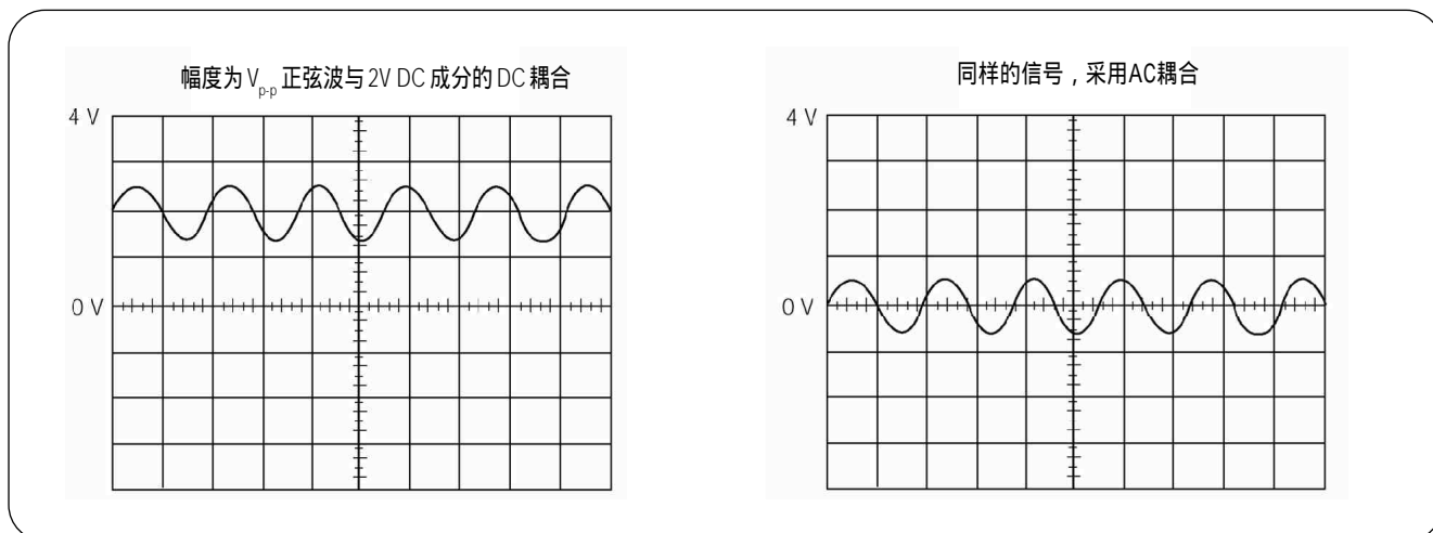
► 图23. AC 和 DC 输入耦合
