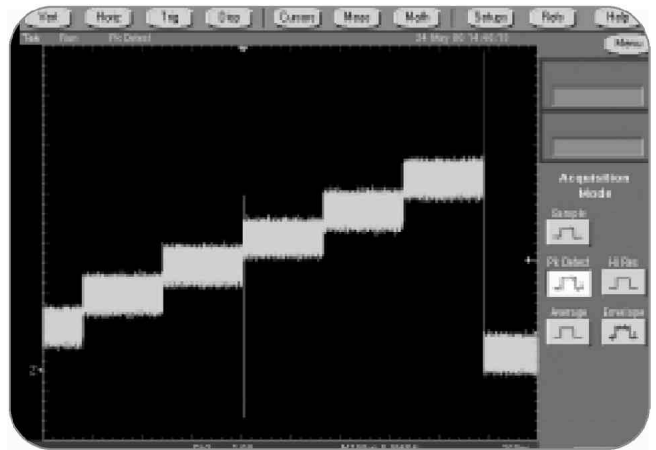
▶ 图27. TDS7000系列示波器采用峰值检测模式能够捕获窄到100ps的瞬态异常
