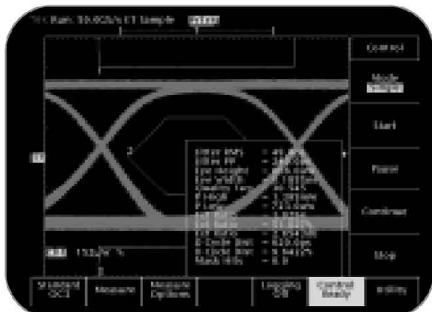
► 图57. TDS700系列示波器配置TDSCEM应用模块，对通信信号进行模板测试。
